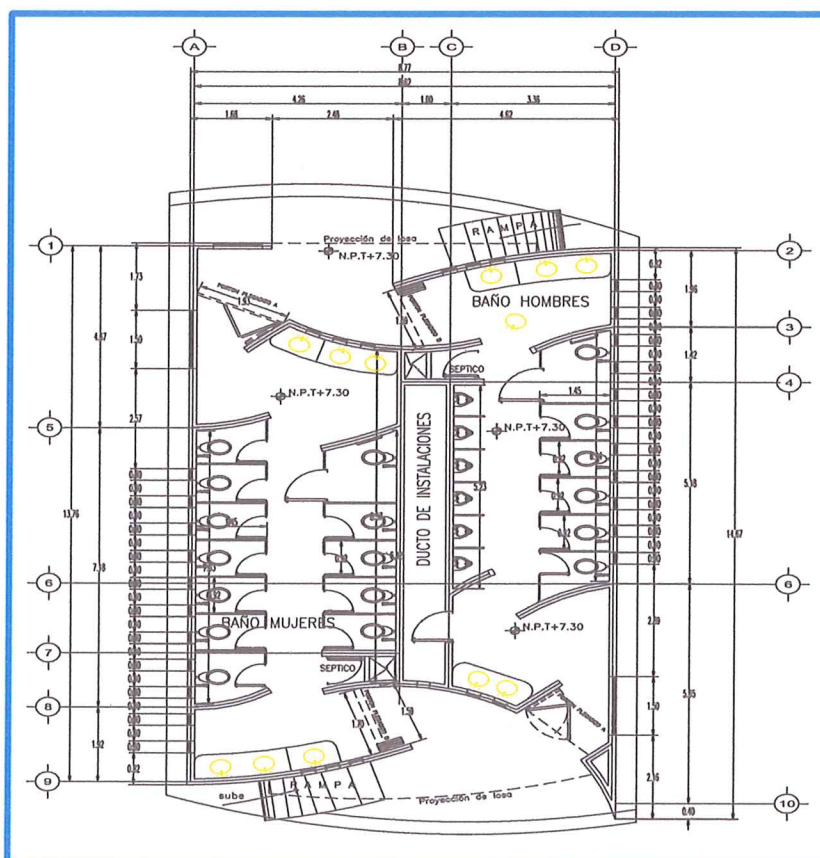
PLANTA ARQUITECTÓNICA BAJA
