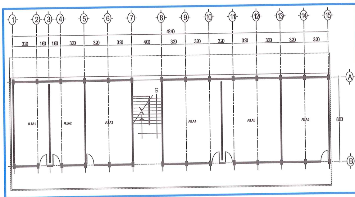
PLANTA ARQUITECTÓNICA ALTA
