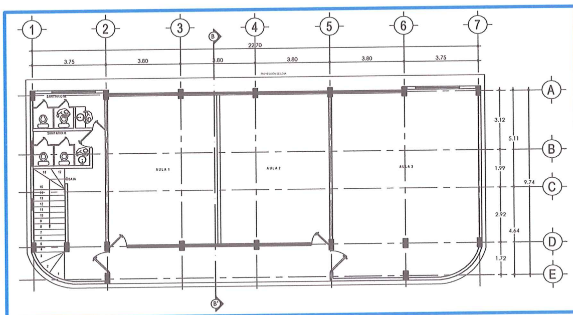
PLANTA ARQUITECTÓNICA 2DO. NIVEL
