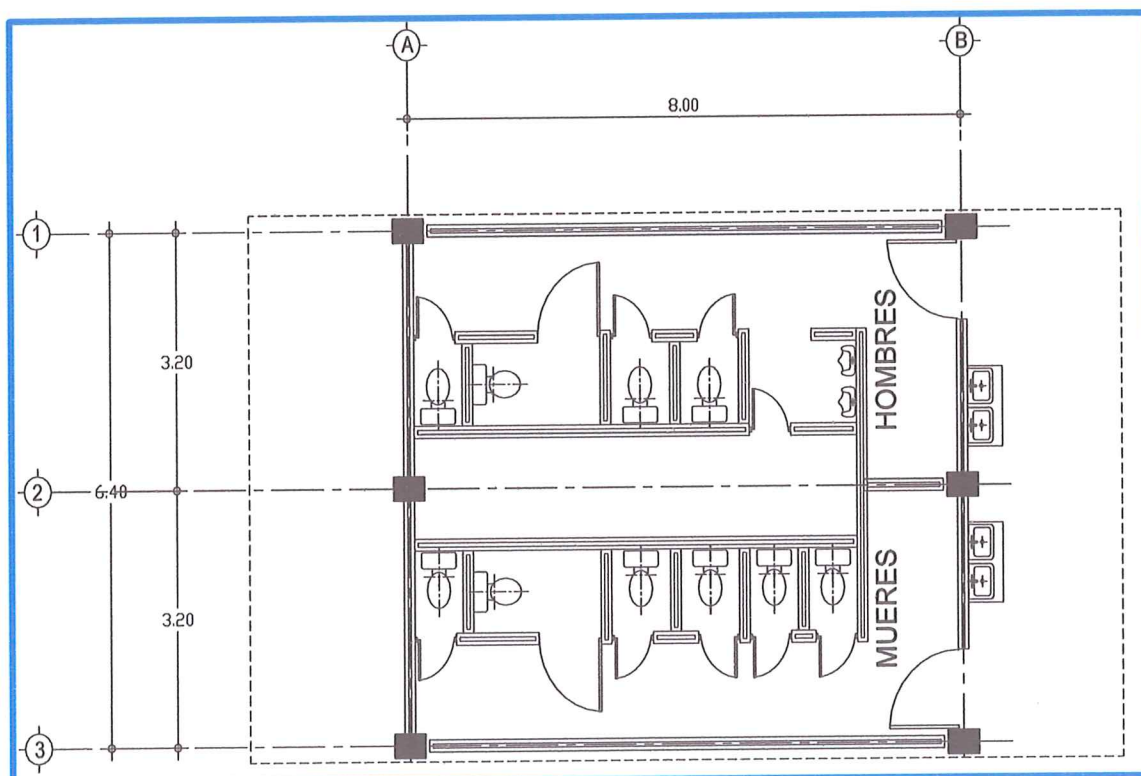
PLANTA ARQUITECTÓNICA BAJA
