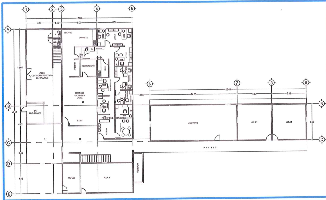
PLANTA ARQUITECTÓNICA BAJA
