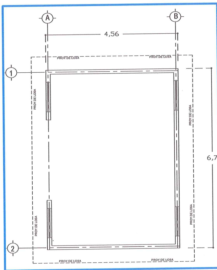
PLANTA ARQUITECTÓNICA DE SUBESTACIÓN ELÉCTRICA
