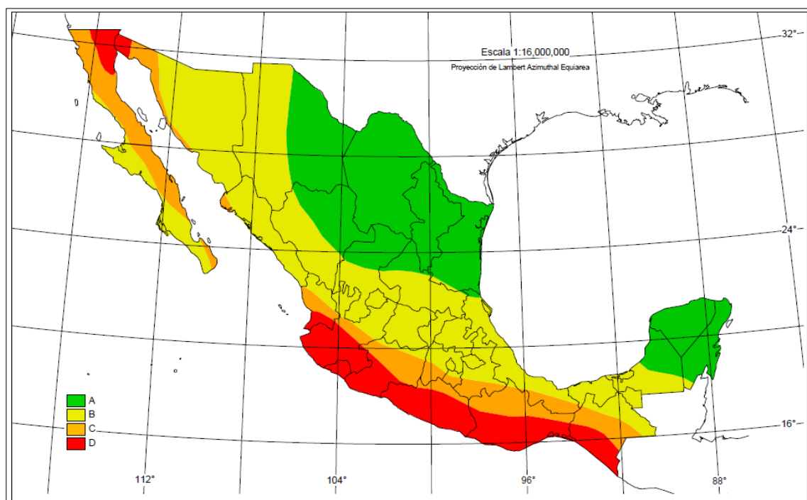
Regionalización Sísmica. Fuente: CENAPRED
