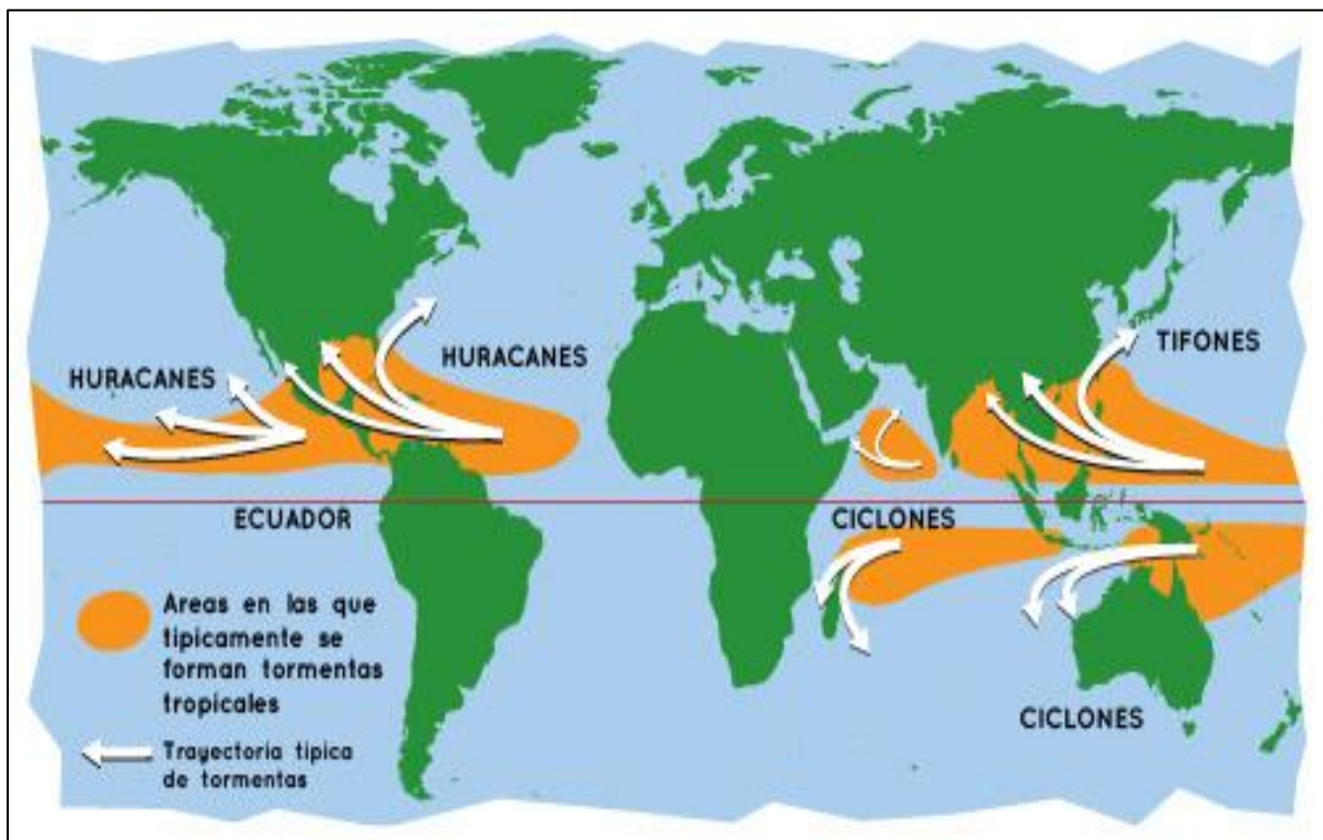
Zonas de Formación de Huracanes. Fuente: https://spaceplace.nasa.gov/hurricanes/sp/
