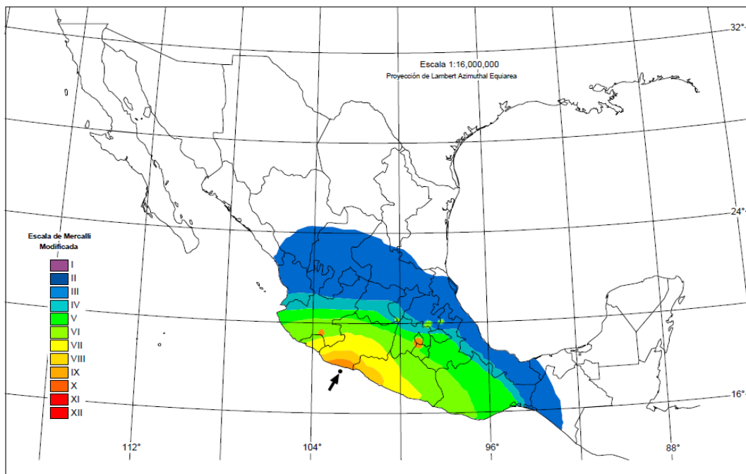
Intensidades Sísmicas. Fuente: CENAPRED
