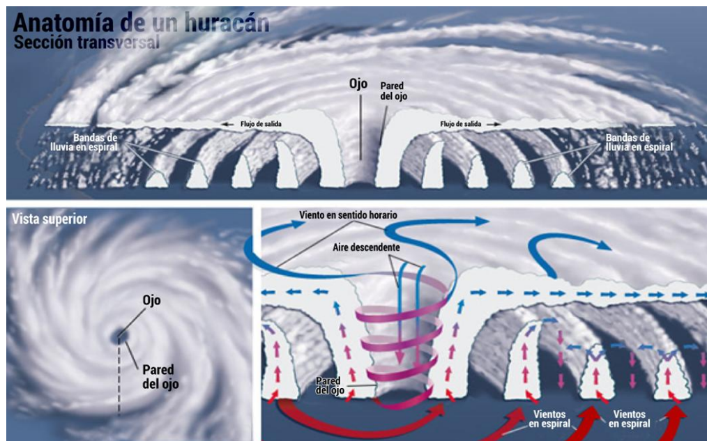
Formación de un Huracán. Fuente: http://bsigeonet.com.mx/news/news-post-temporada-de-huracanes-mx.html
