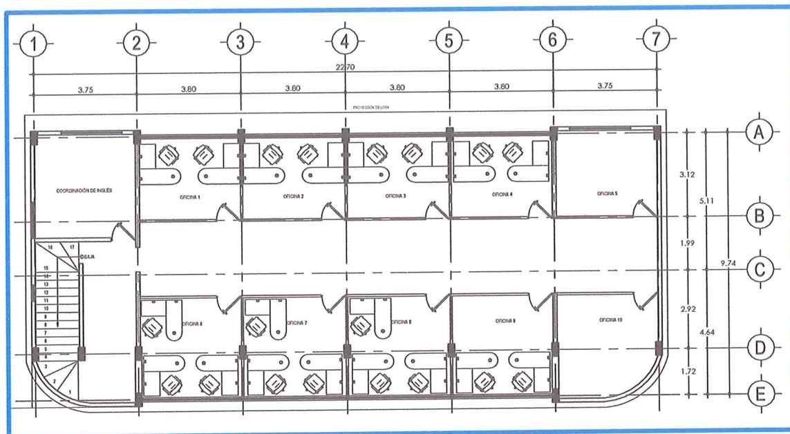
PLANTA ARQUITECTÓNICA 1ER. NIVEL
